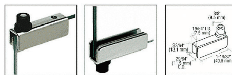
TOP HINGE
